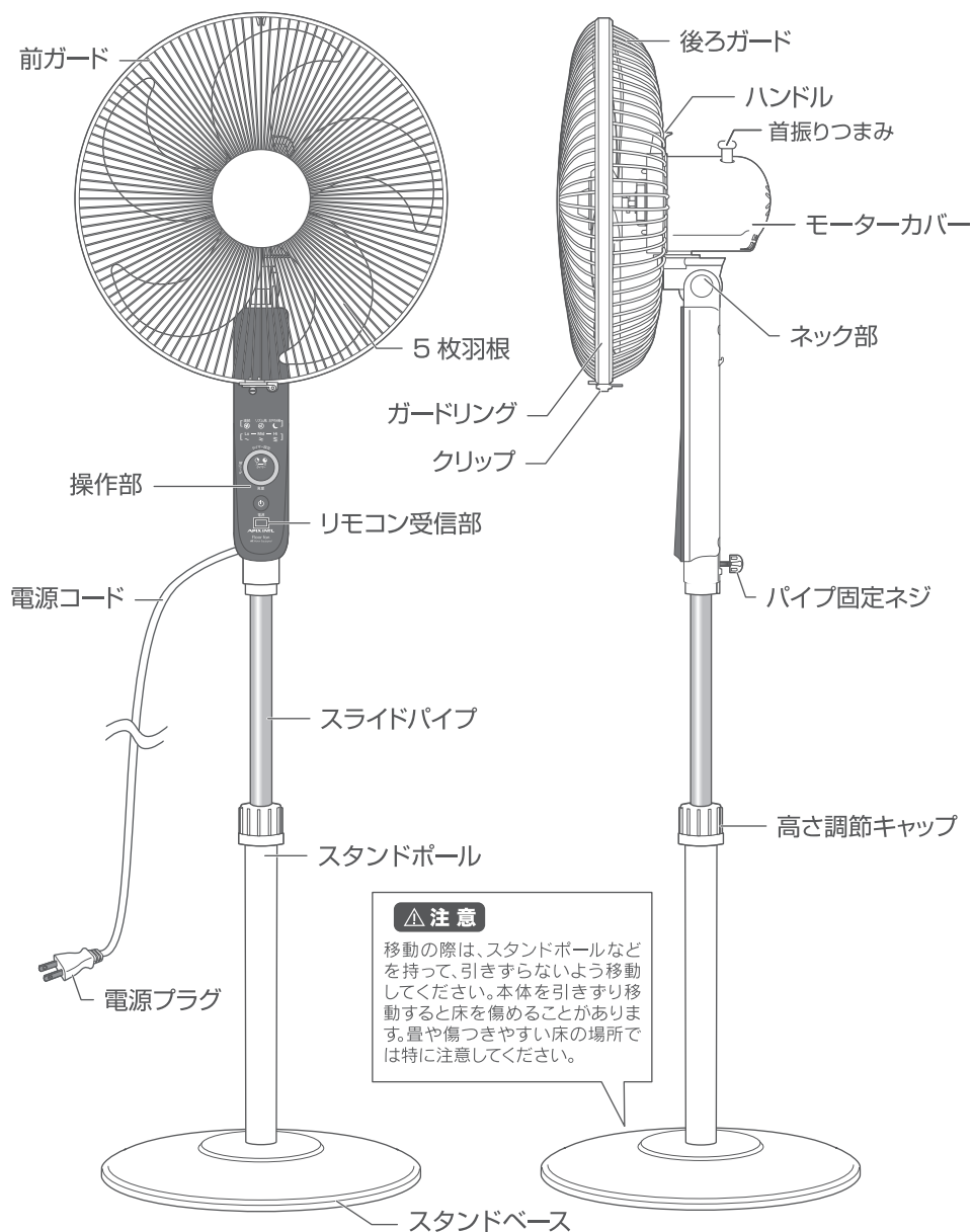
正面図
