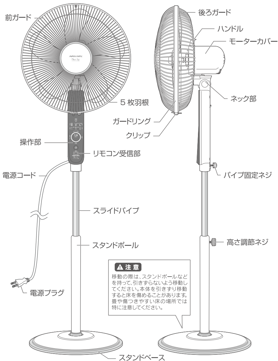
正面図
