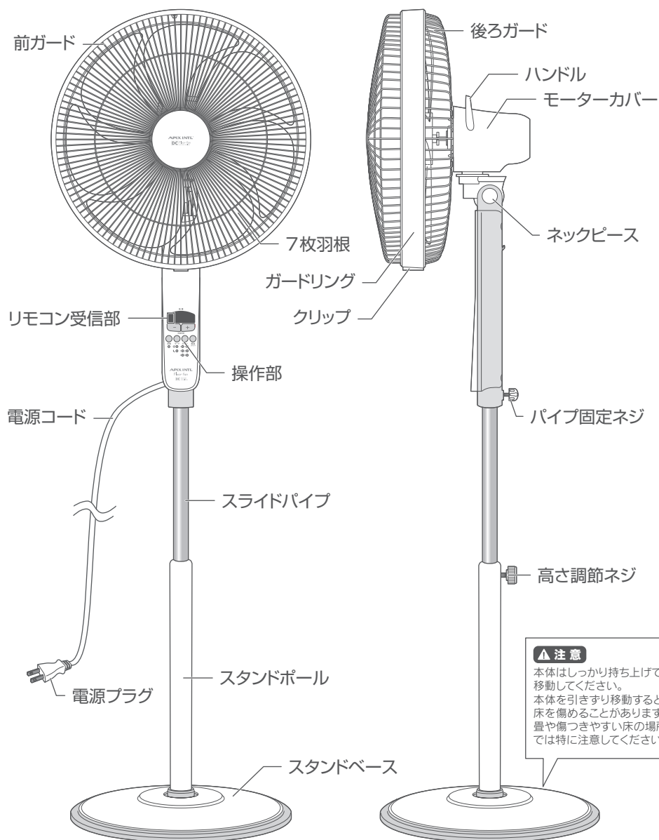
正面図
