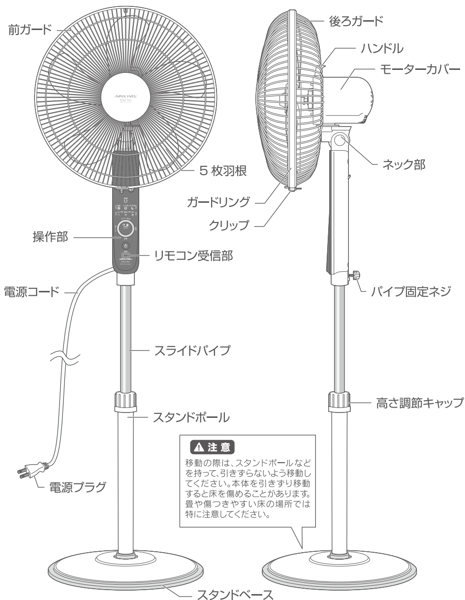
正面図
